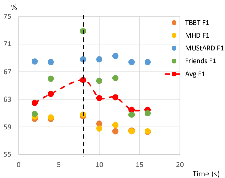
(a) FunnyNet-W V: F1 VS Time windows
