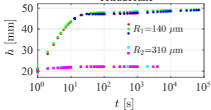
Pentadecane
