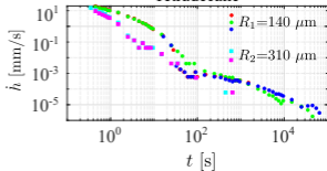
Pentadecane
